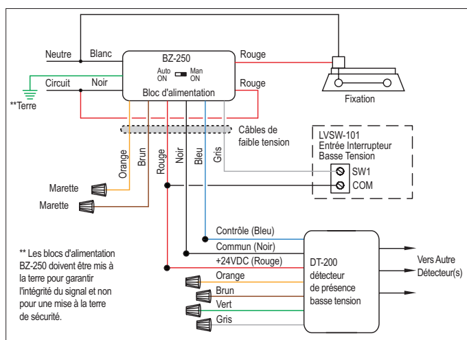
Câblage de la marche manuelle avec un interrupteur instantané basse tension
