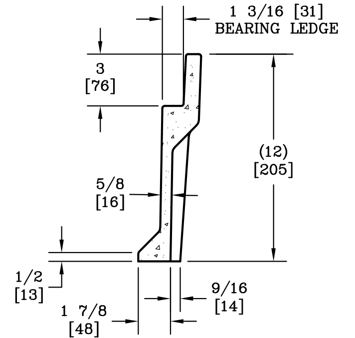
SECTION A-A SCALE: 2"=1' 6 PLACES
