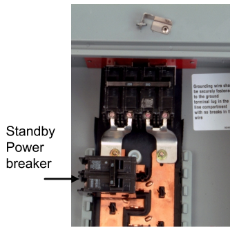
FIG. 2 Install Interlock
