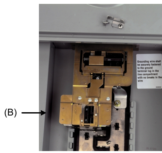
FIG. 2 Install Interlock
