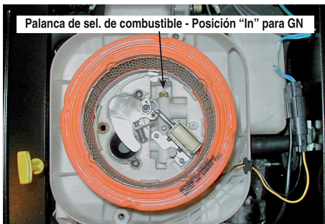
Figura 1.8 - 14, 17, y 20kW, GT-990/GT-999 (cubierta de caja de aire retirada)
