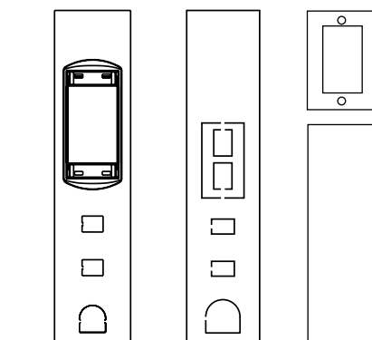
30TC-3S2 (with adapter installed) (avec adaptateur installé) (con el adaptador instalado)
