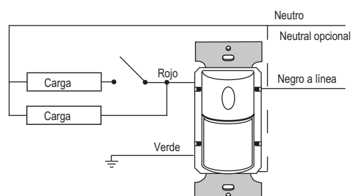
Cableado de iluminación manual de dos niveles
