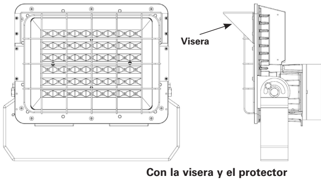
Con la visera y el protector Figura 5
