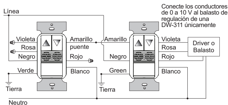
Cableado típico de múltiples vías (DW-311 o DW-311-347 – hasta 4 sensores)
