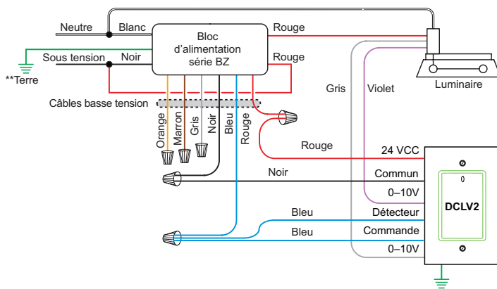
Schéma de câblage 0-10 V
